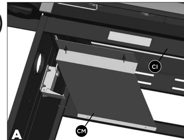
A Vue de l'avant
